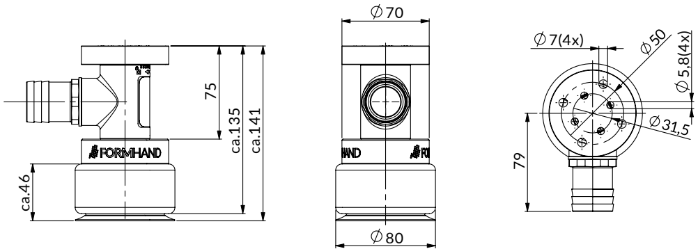
Abbildung: Ansichten des FORMHAND-Modul FH-R80 in der Standardkonfiguration Illustration: Views of FORMHAND-Module FH-R80 in standard configuration
